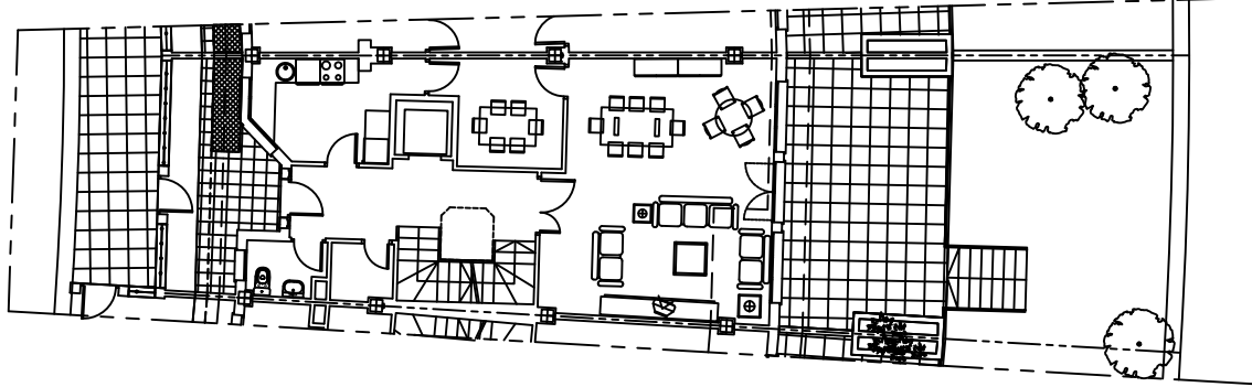
PLTA. BAJA
